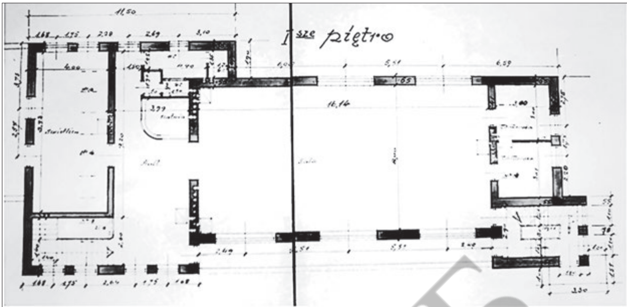
Рис. 1. Польський Народний Дім в Деражно Костопільського повіту Волинського Воеводства. Арх. Едвард Войтович, інж. Павло Дуткевич [4].
