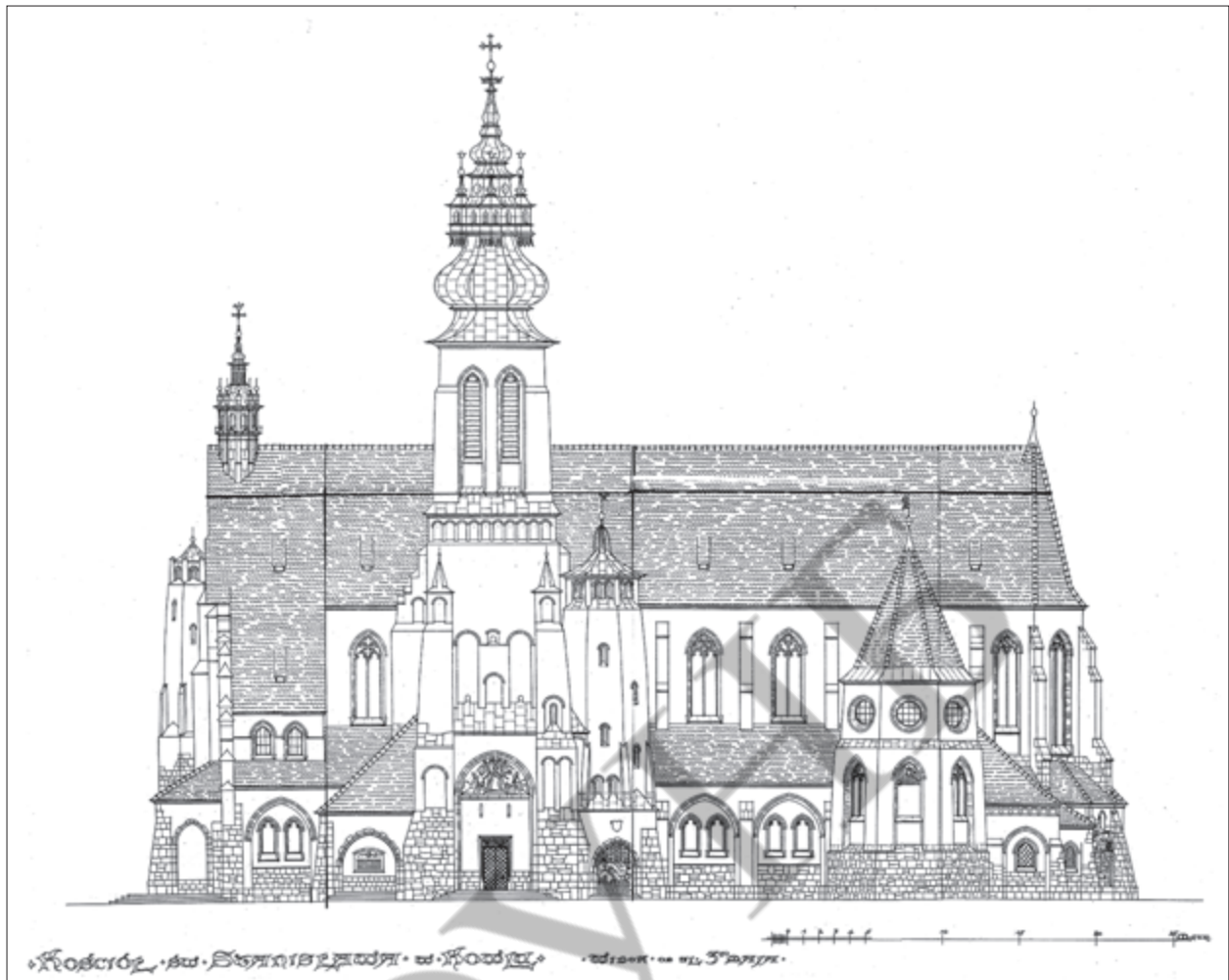
Рис. 3. Ковель. Костел Св. Станіслава. Північно-західний фасад. Арх. С. Шиллер, В. Кононович. Проект, 1924 р.
