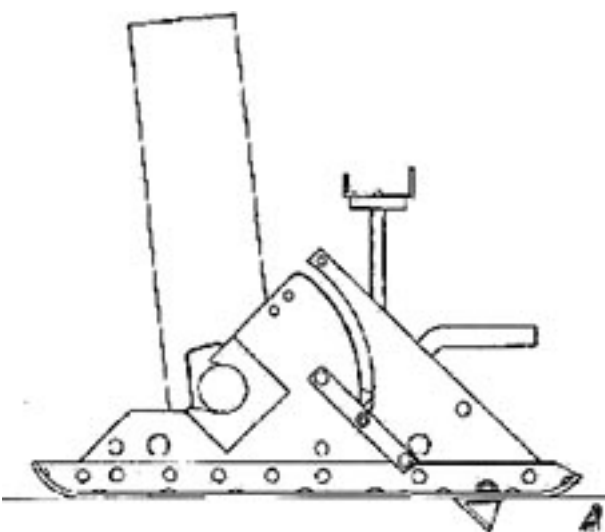
6-дм (152-мм) окопна мортира зр. 1915 г. системи Металевого заводу.
