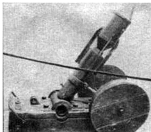
58-мм міномет ФР на дерев'яному станку і його міна.
