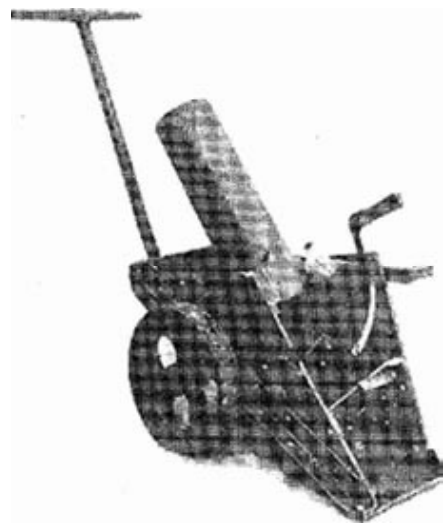
6-дм (152-мм) окопна мортира зр. 1915 г. системи Металевого заводу.
