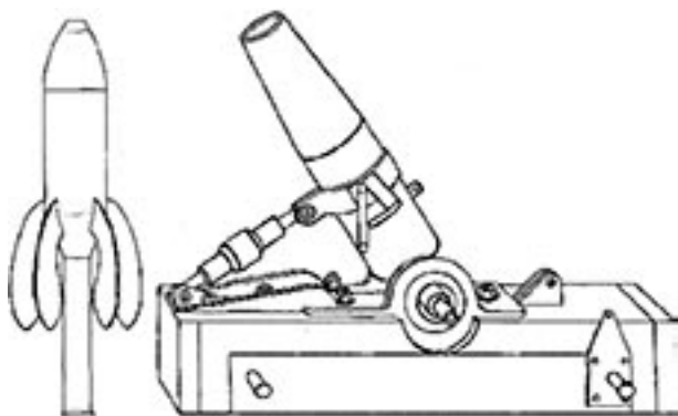
58-мм міномет ФР на дерев'яному станку і його міна.
