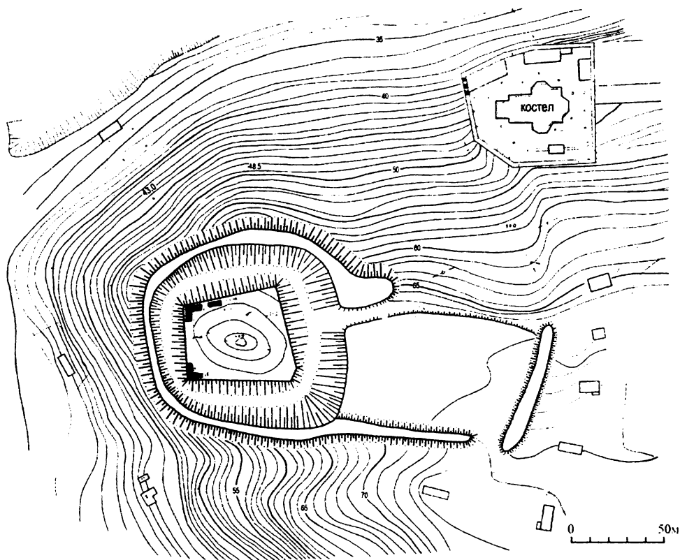
Рис. 7. План замку в с. Тайкурах.
