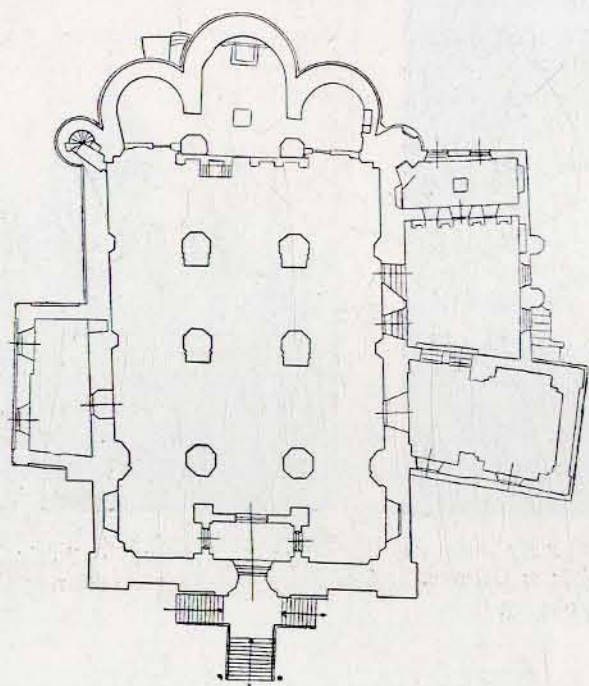
Tow. op. nad Zab. Przesł. Ryc. 34. Wilno. — Cerkiew św. Trójcy. Rzut poziomy.
