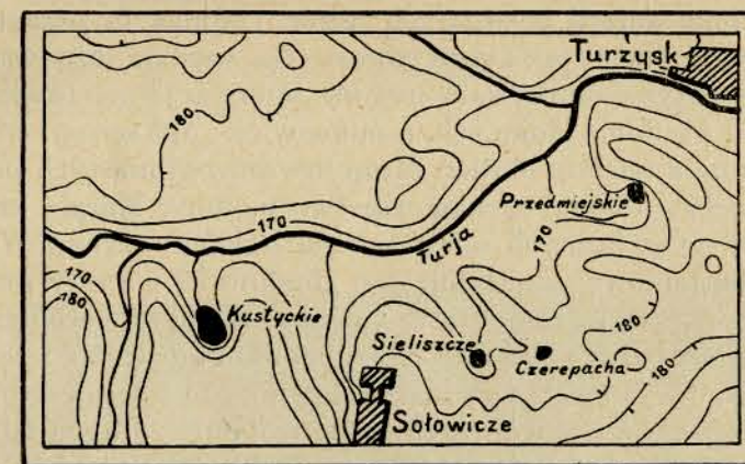
Ryc. 42. Mapa powierzchni poddyluwjalnej okolicy Turzyska 1) . Podziałka 1:100 000 poziomice podłoża co 5 m.
