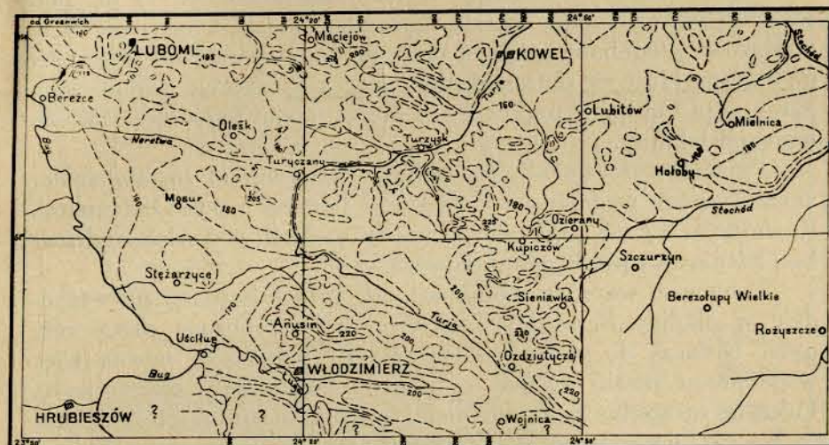
Ryc. 38. Mapa powierzchni poddyluwalnej zachodniej części Polesia Wołyńskiego 1) .
