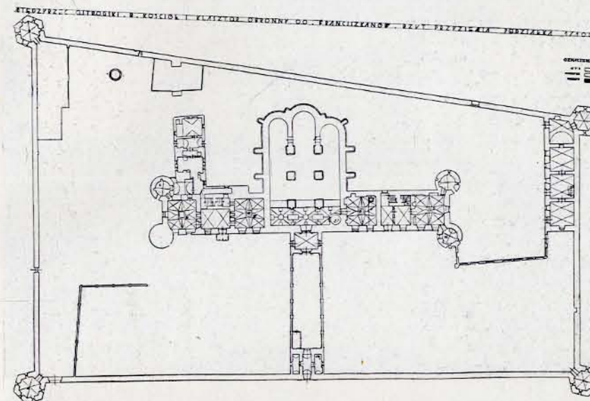
Ryc. 11. Międzyrzecz Ostr. — Klasztor pofranciszkański. Rzut przyziemia.
