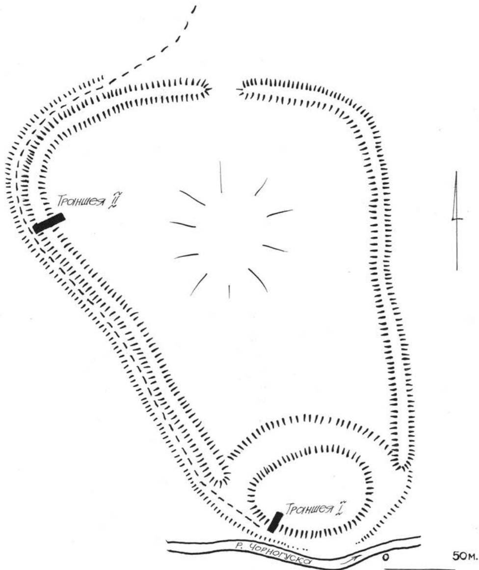
Рис. 1. План Коршівського городища. Fig. 1. Scheme of Korshiv hill-fort.
