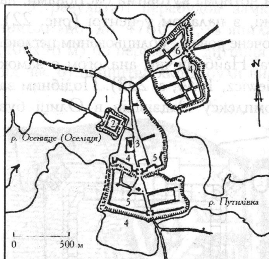
Рис. 23: План укріплень Олики у XVI—XVII ст. (на основі Б.Колоска): 1—фортеця з бастіонами (1558—1567); 2—палац Радзівілів; 3—косяол Св.Трійці в середньому місті; 4—вали навколо міста С. Радзівіла; 5—мури А. Радзівіла навколо Завороття (1630-ті рр.); 6—Луцька мурована брама на Залісочому.
