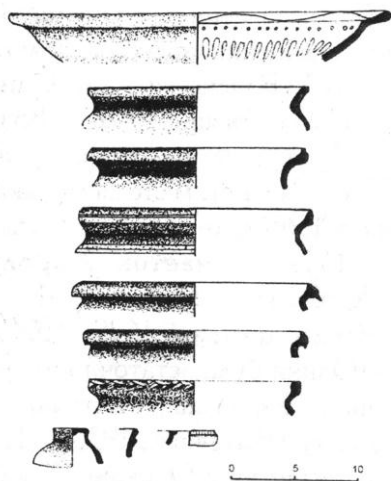
Рис. 16: Дідичі. Гончарний посуд кін. XIII—XV ст.
