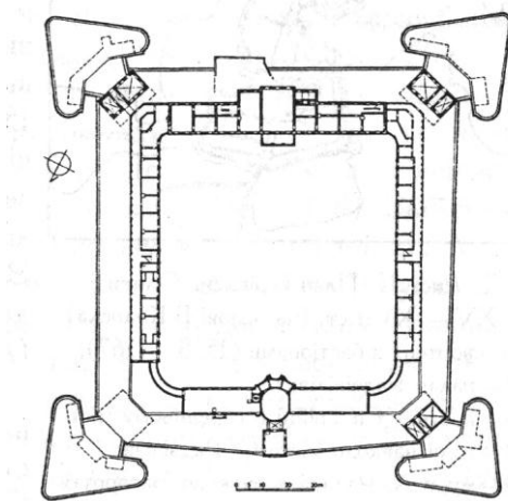
Рис. 22: План замку Олики за Tomkowiicz S.
