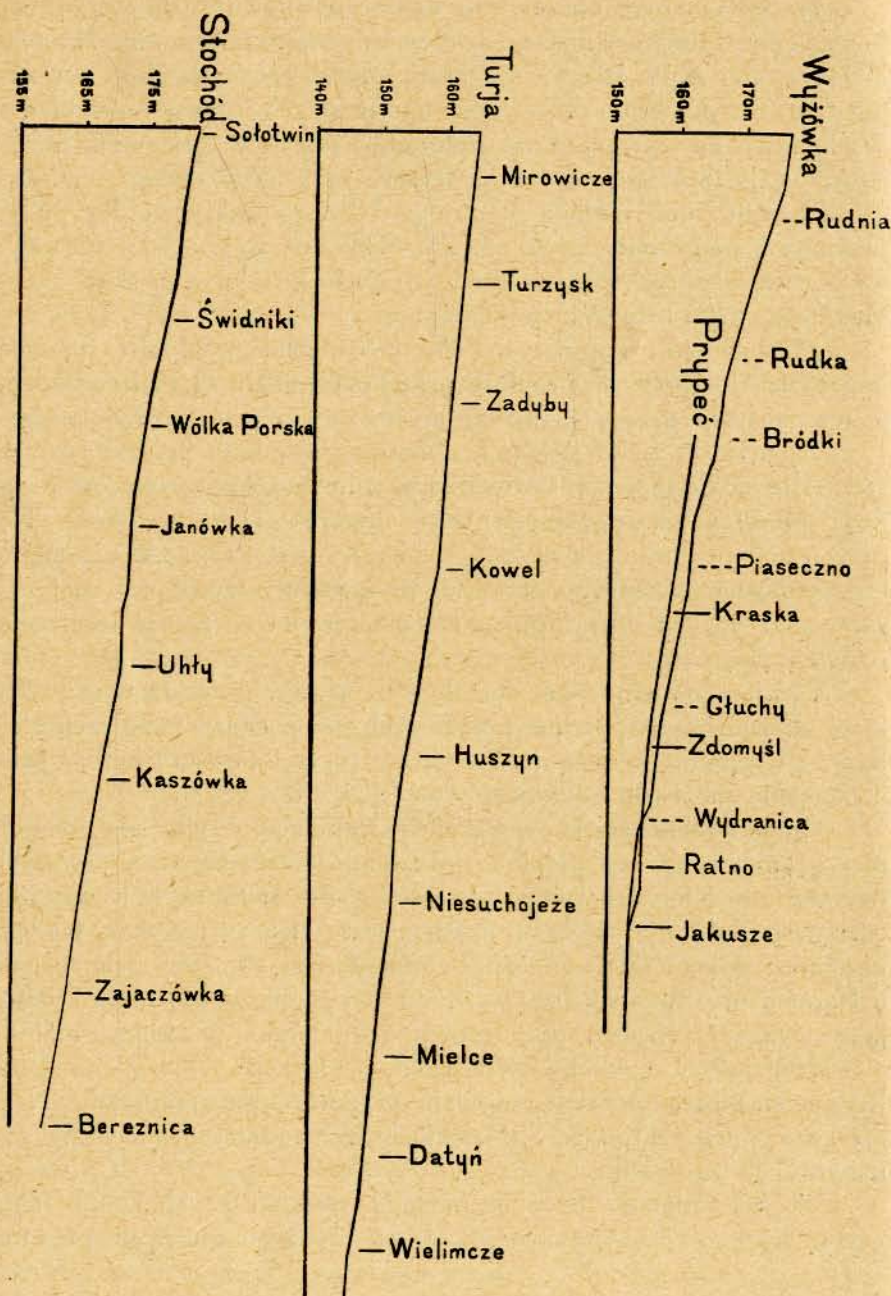
Rys. 39. Profile podłużne rzek powiatu kowieńskiego. Podziałka pozioma 1:700 000, pionowa 1:1100.
