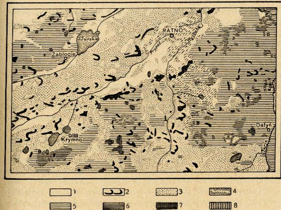
Rys. 31. Schematyczna mapka geologiczna okolicy Ratna.
