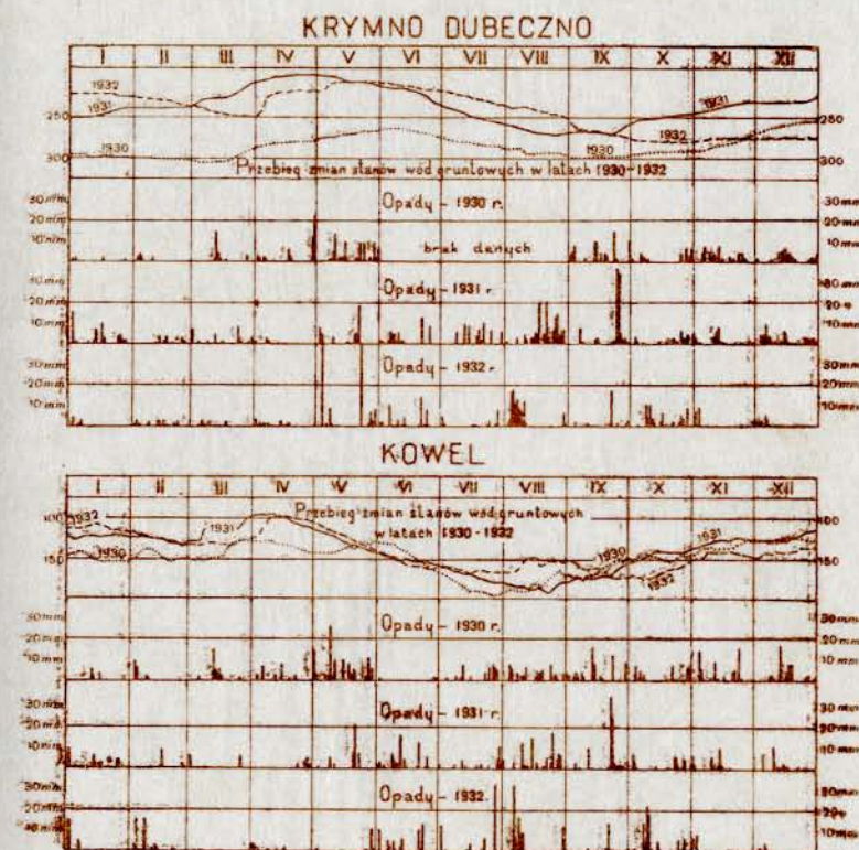
Rys. 41. Przebieg zmian stanów wód gruntowych i opady w latach 1930—1932 w Kowlu i Krymnie Dubecznie.
