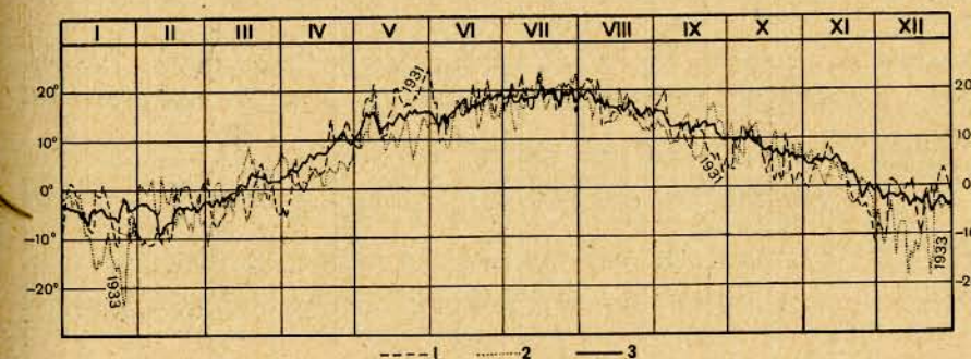
Rys. 49 Wykres dziennych temperatur w Powórku w roku 1931 i 1933 oraz średnich dziennych temperatur z okresu 1930—1936 r.
