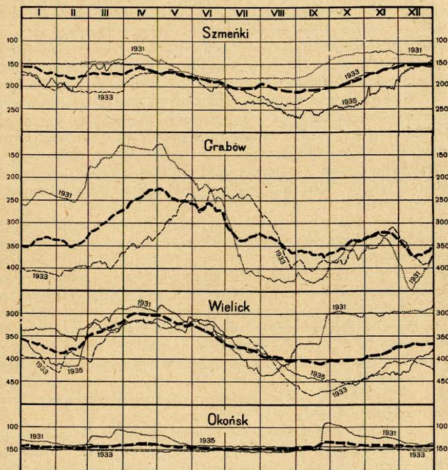
Rys. 45. Przebieg zmian stanów wód gruntowych w 1931, 1933 i 1935 roku i średnia dzienna okresu 1931 — 1935 r. (linja gruba przerywana).
