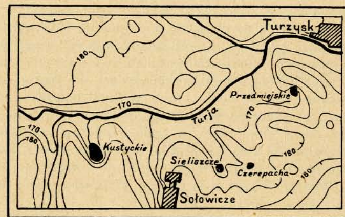
Rys. 48. Mapka powierzchni poddyluwalnej okolicy Turzyska.
