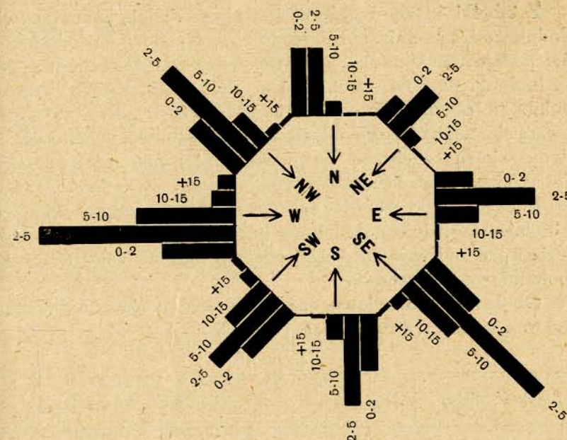
Rys. 53. Kierunki i szybkość wiatrów w Powórku w okresie 1930—1936 r. Cyfry ponad słupkami — szybkość wiatru w metrach na sekundę.
