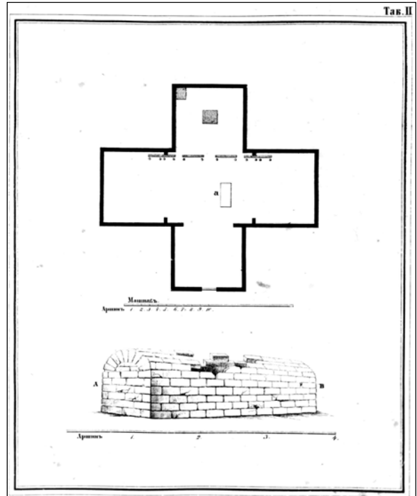
Рис. 2. План Свято-Троїцької церкви біля с. Вербки (за М. Д. Іванішевим)
