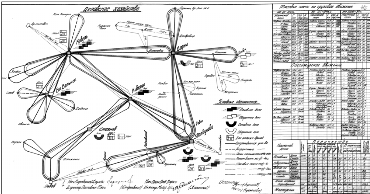
План відновлення деповського господарства Ковельської залізниці на 1946—1950 рр. (Держархів Волинської області, Р-3165, Управління Ковельської залізниці, 1940—1941, 1944—1953 роки, оп. 5, спр. 20, арк. 11)
