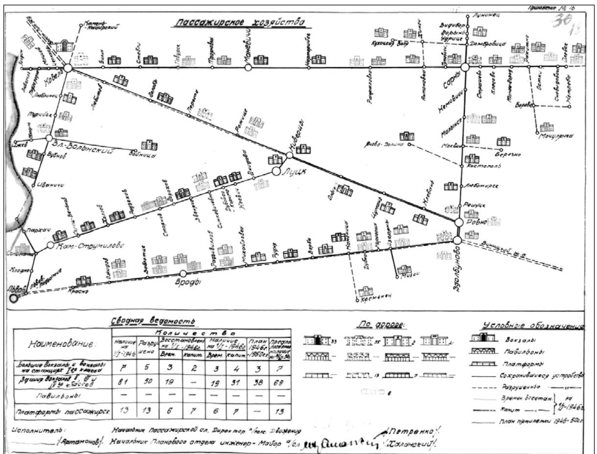
План відновлення пасажирського господарства Ковельської залізниці на 1946—1950 рр. (Держархів Волинської області, Р-3165, Управління Ковельської залізниці, 1940—1941, 1944—1953 роки, оп. 5, стр. 20, арк. 18)
