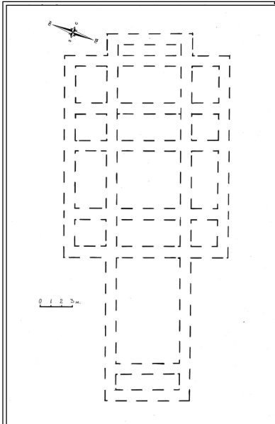
Рис. 5. План залишків фундаменту Свято-Троїцької церкви біля с. Вербки (за Ю. М. Мазуриком)
