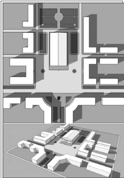
Рис.1. Варіант планування №1, розроблений «ДІПРОМІСТО» Модель реконструкції (виконали: Ковальчук Р., Омельчук І.)
