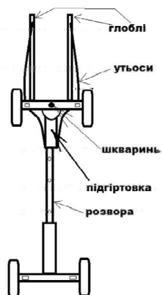
2. Схема воза. Малюнок автора.
