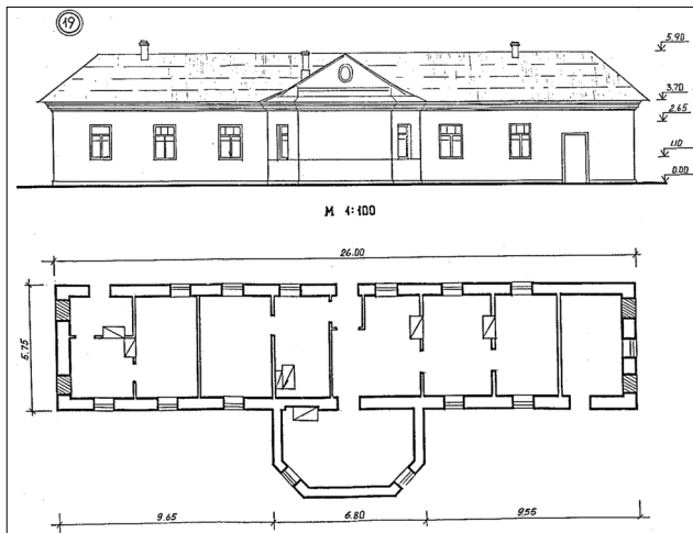
Рис. 3. Схематичний обмір будинку колишньої плебанії (1993 р.).
