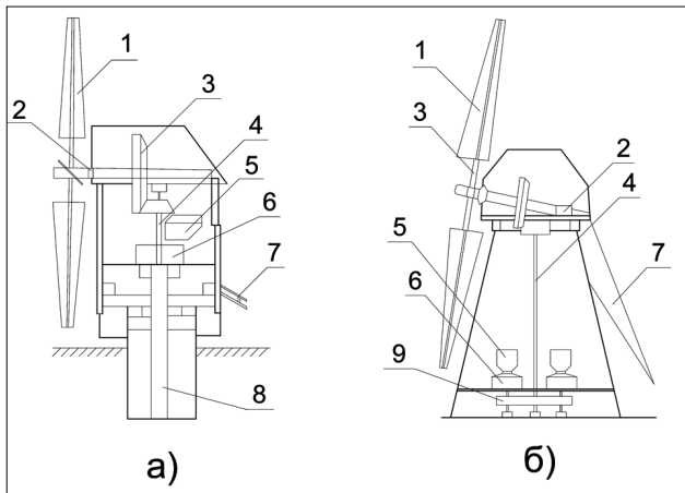
Рис. 4. Схеми козлових (а) і шатрових млинів (б): 1 – вітроколесо; 2 – головний вал; 3 – одноступінчата передача; 4 – вал жорна; 5 – засипний лоток; 6 – жорно; 7 – водило; 8 – центральний стовп; 9 – двоступінчата передача. Опрацьовано автором за «Енергетика...»
