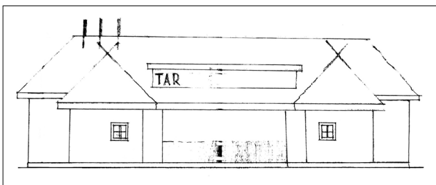
Рис.8. Вхідний павільйон. Фасад зі сторони території виставки.
