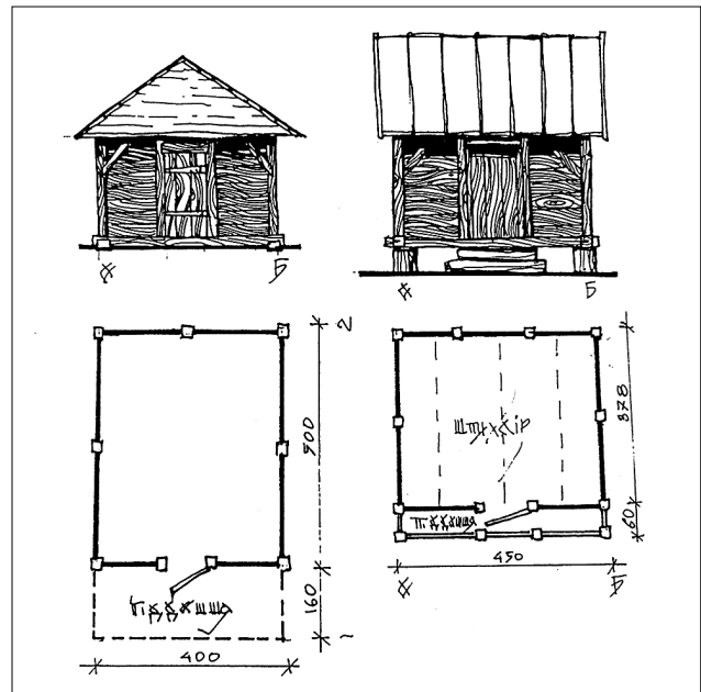
Рис. 8. 1 – Шпихлір поч. XX ст. зі с. Федорівців Сокальського р-ну Львівської обл.; 2 – Шпихлір поч. XX ст. зі с. Луциць Сокальського р-ну Львівської обл.
