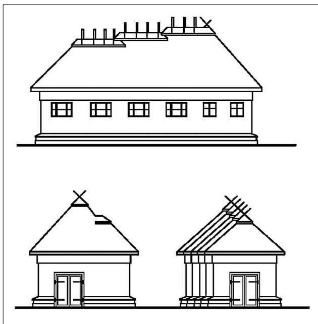
Рис. 15. Павільйон №2. Головний та бічний фасади. Прорис проекту поч.1930-х рр.
