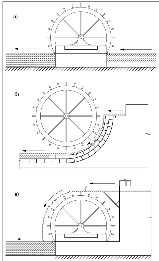
Рис.2. Системи подачі води на колесо: а) нижньобійнє; б) середньобійнє; в) верхньобійнє. Креслення автора.
