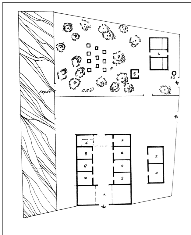
Рис. 4. Двір з «підварком» кін. XIX – поч. XX ст. зі с. Вузлого (присілок Підгайок) Радехівського району Львівської обл. 1 – хата; 2 – хлів; 3 – стодола; 4 – піддашня-шопа; 5 – майстерня; 6 – січкаря; 7 – шопа; 8 – шпихлір; 9 – пасіка; 10 – криниця
