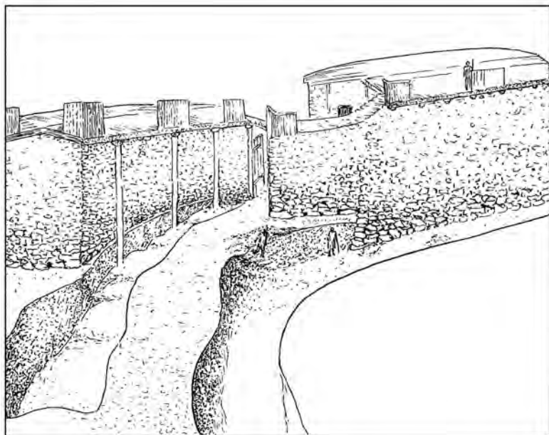
Рис. 1.11. Реконструкція Левенцівської та Каратаївської фортець: 1 – загальний вигляд з навпільного боку (з півночі); 2 – вигляд зі сходу ділянки Левенцівської фортеці зі спорудами та ровами 1–7; 3 – частина з ланками 5–6 та проїздом (за С. Братченком)
