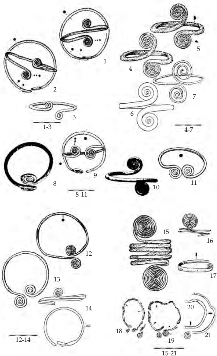
Рис. 1.41. Браслети зі спірально закрученими кінцями з території України (за С. Лисенко)
