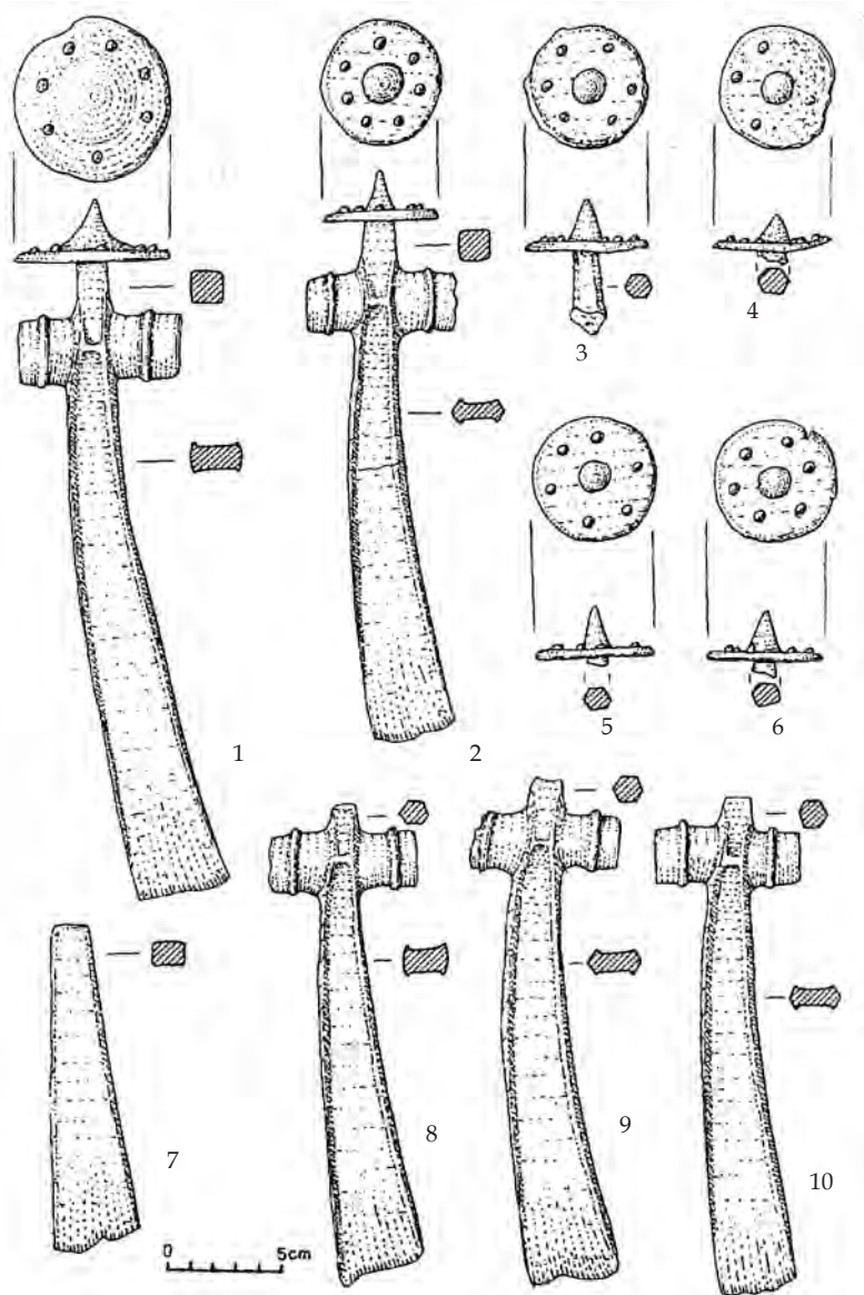
Рис. 4.20. Скарб чеканів з щитоподібним обухом з Квасови (Закарпаття, Україна) доби пізньої бронзи (за Й. Кобалем, 1997)
