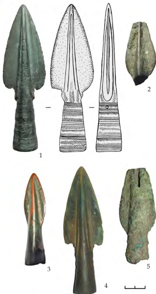
Ил. 53. Наконечники списів пізньої доби бронзи: 1 – с. Піддубці Луцького р-ну; 2 – с. Боратин Луцького р-ну; 3 – Острозький р-н Рівненської обл.; 4 – Любомльський р-н Волинської обл. (фонди ЛКМ); 5 – Горохівський р-н Волинської обл. Фото І. Маркуса, Г. Охріменка
