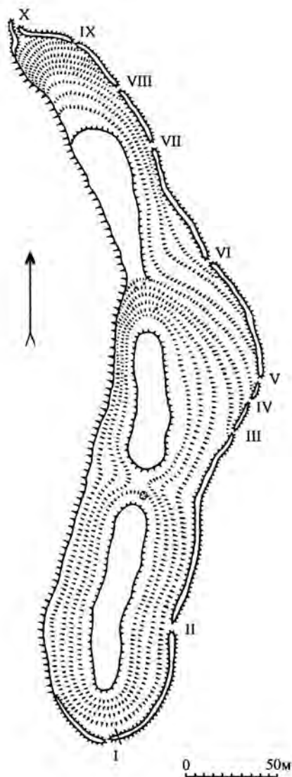
Рис. 1.13. Загальний план городища Шелестово (за Е. Балагурі)
