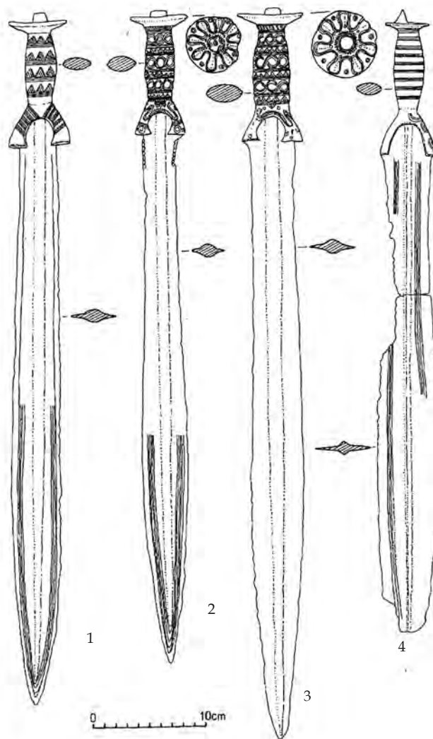
Рис. 4.19. Скарб мечів з Негрова доби пізньої бронзи (Закарпаття, Україна) (за Й. Кобалем, 1997)
