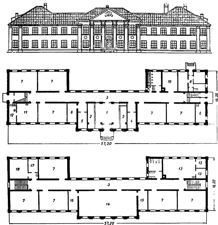
Рис.2. Типовий проект школи на 400 учнів. Архітектор О. Маринченко. Головний фасад та плани 1-го і 2-го поверхів: 1 – вестибюль, 2 – гардероб, 3 – рекреація, 4 – кабінет лікаря, 5 – канцелярія, 6 – кабінет директора, 7 – клас, 8 – кімната сторожа, 9 – квартира директора, 10 – бібліотека, 11 – буфет, 12 – комора буфета, 13 – лабораторія, 14 – гімнастичний зал, 15 – кімната спортивного інвентаря, 16 – роздягальня, 17 – кабінет біології, 18 – учительська
