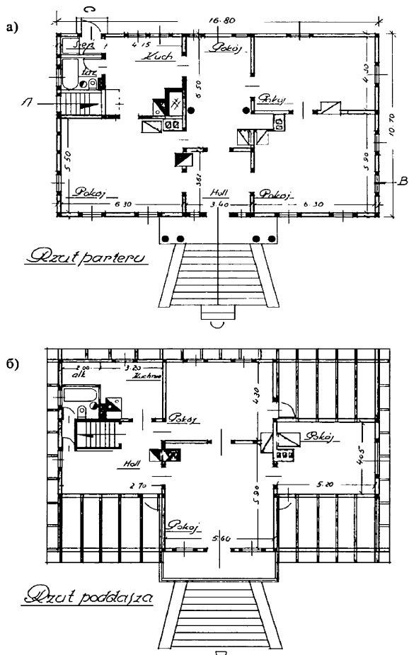
Рис. 7. Житловий будинок у пров. Стрімкому в Кременці. Проект ремонту. Инж. А.Столяров. 1938 р.
