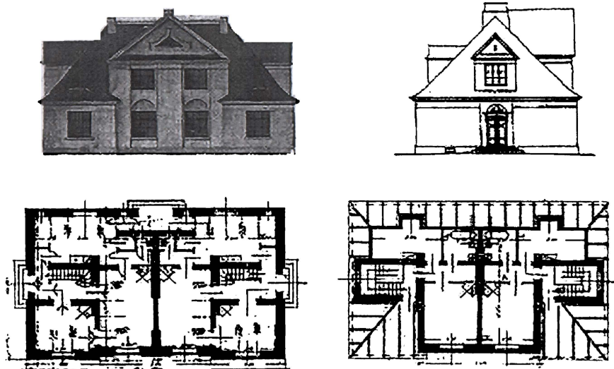
Рис. 7. Проект будинку для 2-х сімей (тип «L»). Арх. Т. Бурше. 1924 р
