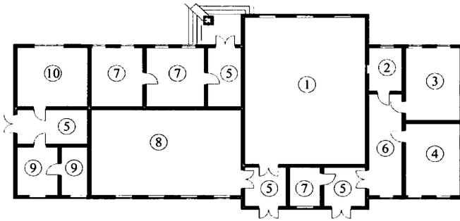
Рис. 2. Планувальна схема вокзалу станції Маневичі: 1) зал очікування; 2) каса; 3) кабінет начальника станції; 4) кабінет чергового по станції; 5) тамбур; 6) коридор; 7) службові приміщення; 8) магазин; 9) медпункт; 10) товарна контора (опрацювання автора)
