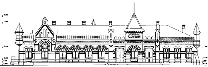
Рис. 1. Головний фасад залізничного вокзалу станції Маневичі. 1904 р. (графічна реконструкція автора)
