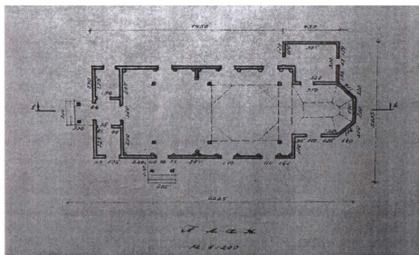
Рис. 6. с. Городнє. План церкви св. Луки, 1961 р.
