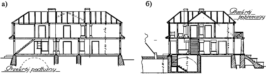
Рис. 8. Житловий будинок у пров. Стрімкому в Кременці. Проект ремонту. Інж. А. Столяров. 1938 р. Графічне опрацювання автора за матеріалами ДАТО. [13]: а) поздовжній перекрій; б) поперечний перекрій.
