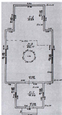
Рис. 21. с. Забужжя. План церкви, 1959 р.
