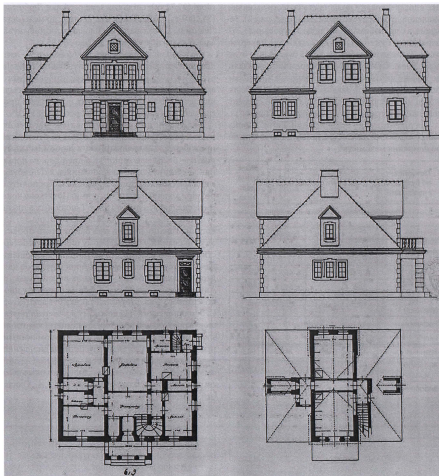
Рис. 6. Проект будинку старости (тип III-R). Арх. А. Ранецький. 1924 р.
