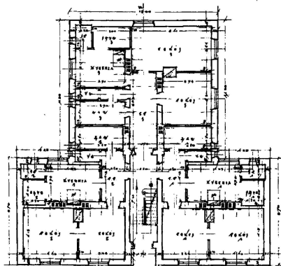
Рис. 4. Проект колонії для службовців. Фасади та плани житлового будинку для 6-ти сімей. Арх. А. Ранецький. 1924 р.
