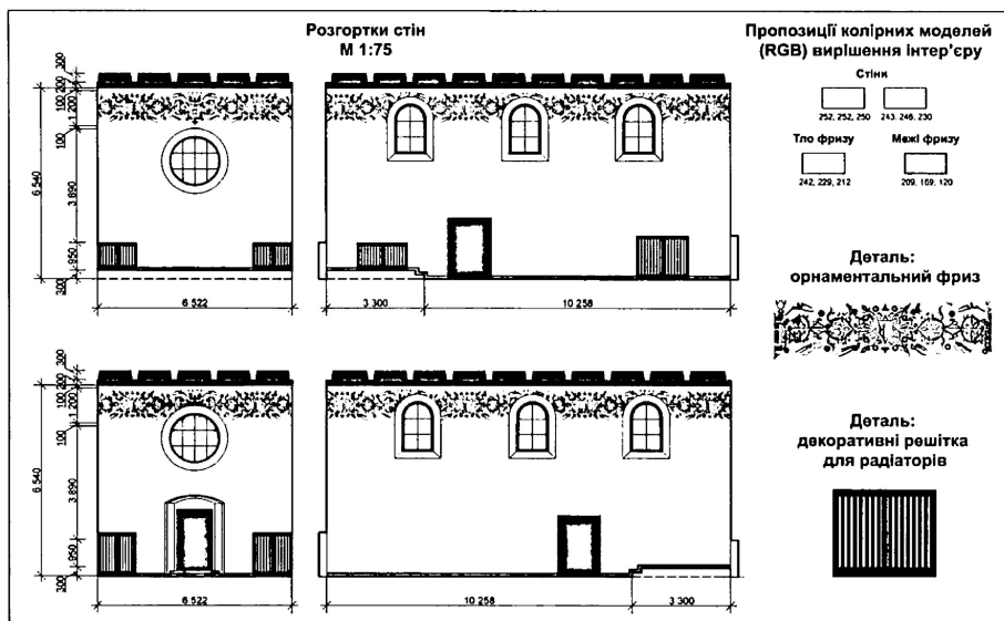
Рис. 1. Проект інтер'єру Тронної зали в замку Острозьких-Любомирських в Дубно. Розгортка стін. Арх. Ю. Ягодка. Консультант д. арх. О. Михайлишин
