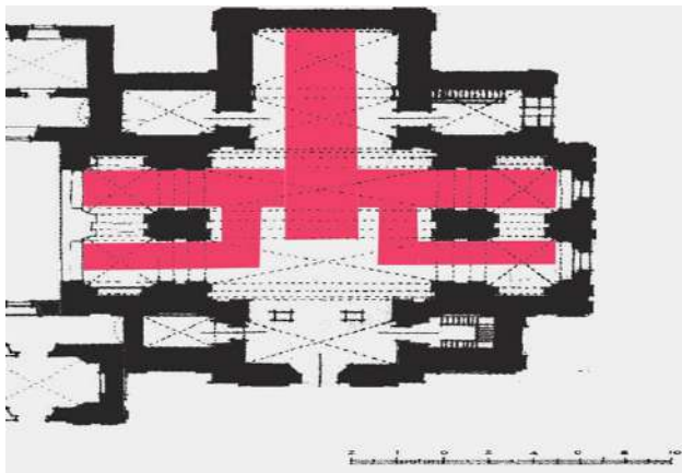
Рис. 7. План підземелля костелу домініканців у Богородчанах (за З. Федунківим)
